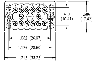
36 PIN RECEPTACLE
