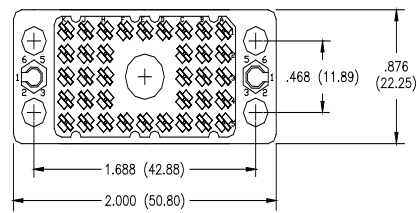
36 PIN RECEPTACLE
